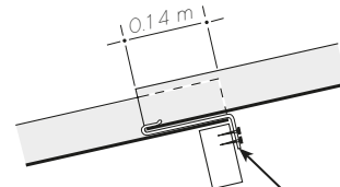
Gancho 55, 150 ó 250 mm. de acuerdo con el tipo de estructura empleada.
